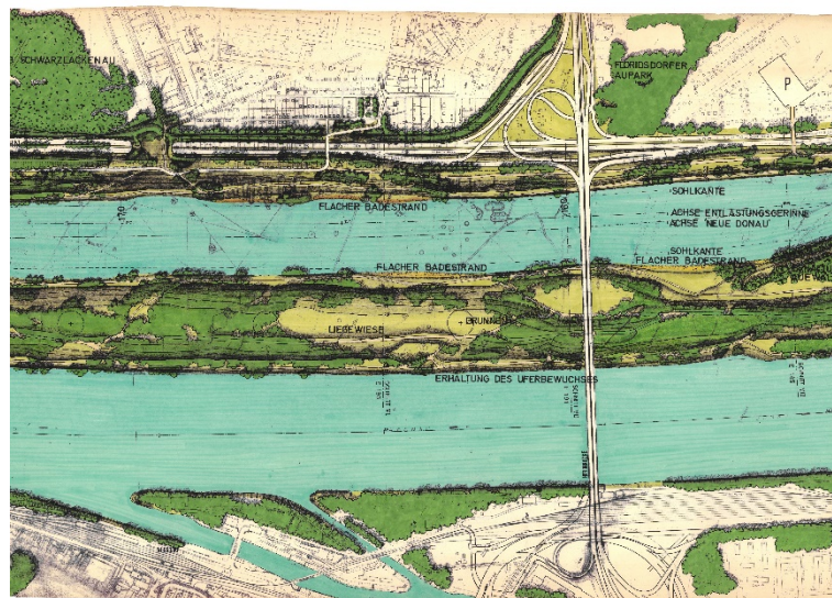
Donauinsel, Entwurf Gottfried und Anton Hansjakob, Wien, 1976; Ausführungsplan Nordteil, Ausschnitt (© LArchiv, BOKU Wien)
